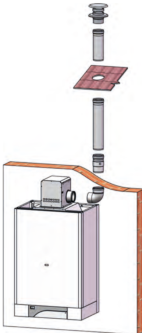
Дымоудаление 1х100 выхлоп (вертик.)
