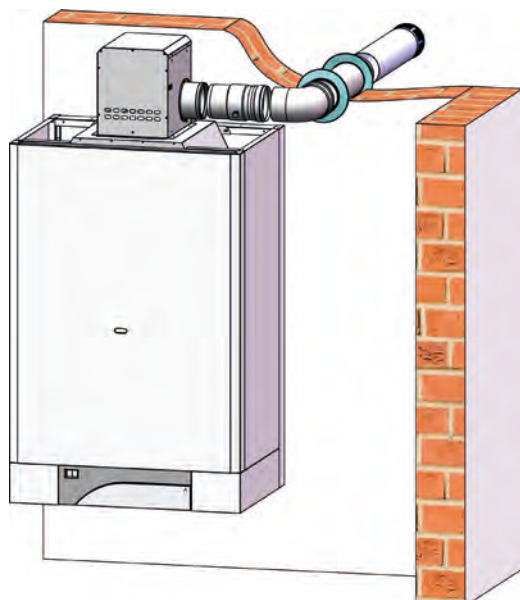
Дымоудаление 1х100 выхлоп (горизонт.)
