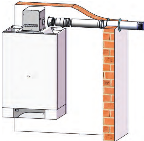
Дымоудаление 1х100 выхлоп (горизонт.)
