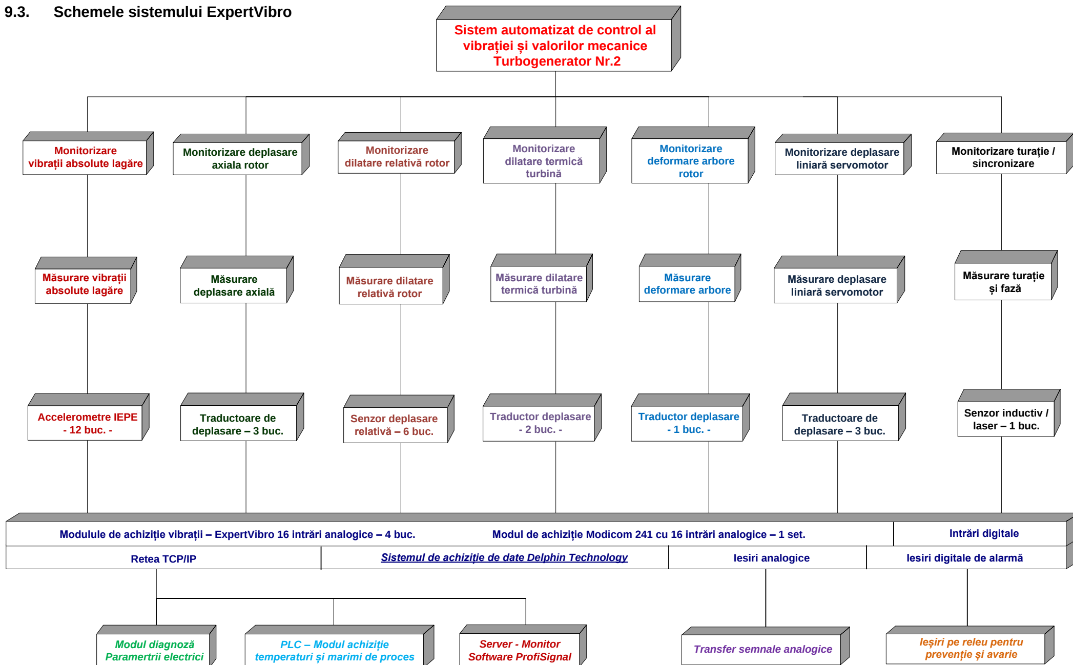
Figura 1. Schema bloc a sistemului
