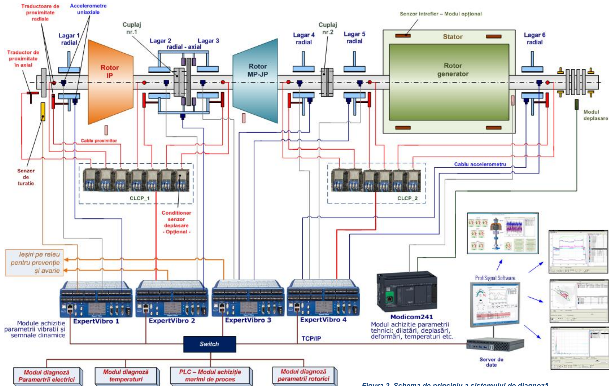
Figura 2. Schema de principiu a sistemului de diagnoză
