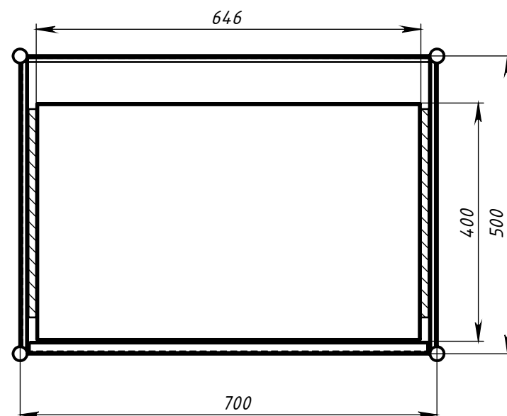
A-A (1 : 9)
