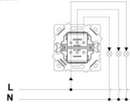
Bağlantı Şeması Connection Scheme Схема Подключения
