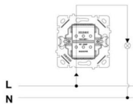
Bağlantı Şeması Connection Scheme Схема Подключения
