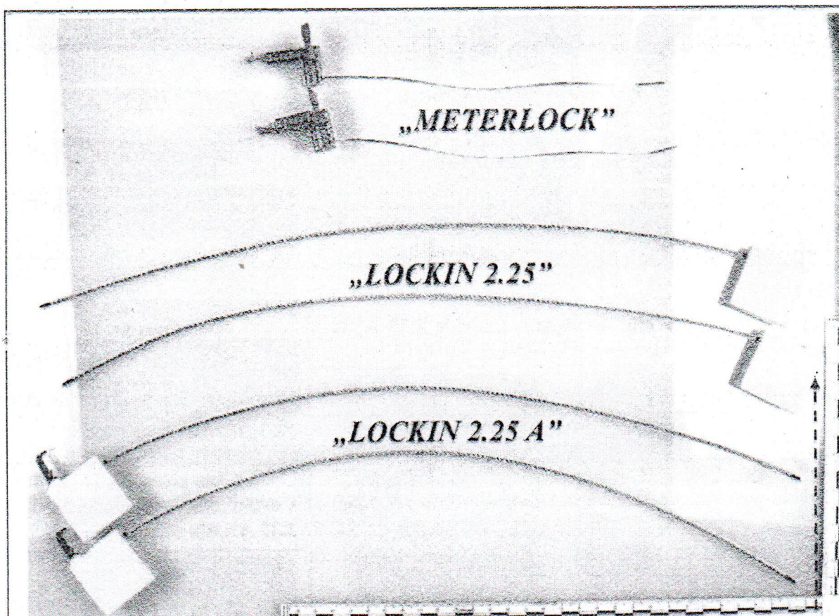
Imaginea nr. 1: Obiectele prezentate spre examinare: două dispozitive de sigilare „Lockin 2.25 A” (1-1149(17)-1/3); două dispozitive de sigilare „Lockin 2.25” (1-1149(17)-2/3); două dispozitive de sigilare „Meterlock” (1-1149(17)-3/3).
