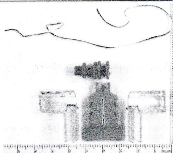
Imaginea nr. 27: Construcția interioară a corpului dispozitivului de sigilare „Meterlock” (1-1149(17)-3/3).
