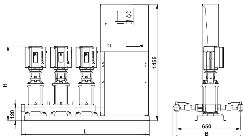
Fig. 14 Schiță dimensională a unui sistem de repompare Hydro MPC cu un dulap de control montat pe aceeași placă de bază ca și pompele (design A)
