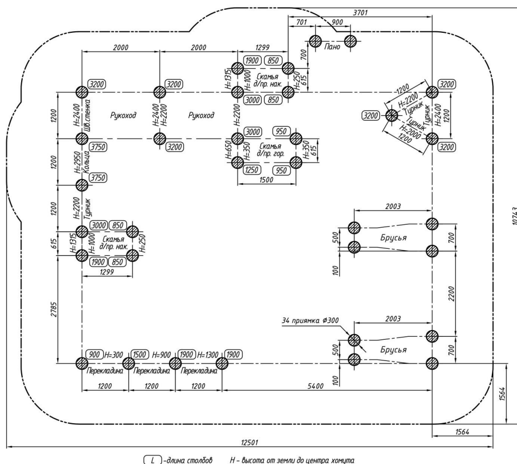
Fig. 3 – Plan de amplasare fundație
