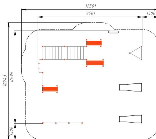
Fig. 1 – Spații de siguranță
