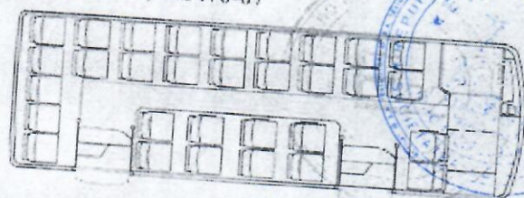
Вариант 2. Количество мест для сидения 31+1 (29 для детей + 2 сопровождающих), пассажировместимость 31
