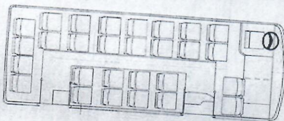
Вариант 2. Количество мест для сидения 28+1, пассажировместимость 46
