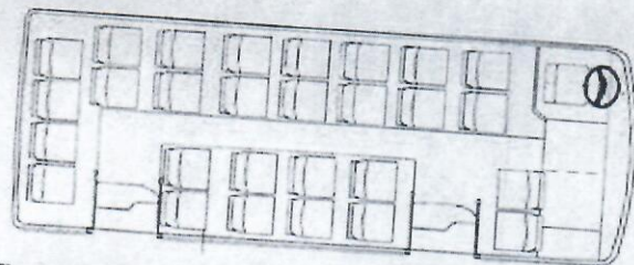
Вариант 2. Количество мест для сидения 28+1, пассажировместимость 46
