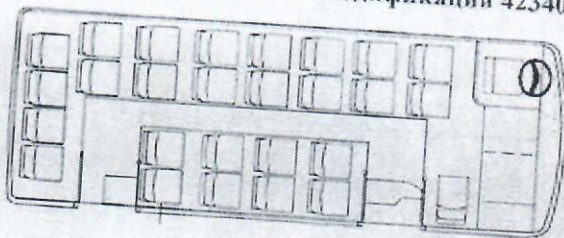
Вариант 1. Количество мест для сидения 27+1, пассажировместимость 45
