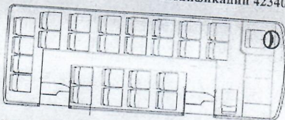
Вариант 1. Количество мест для сидения 27+1, пассажировместимость 45
