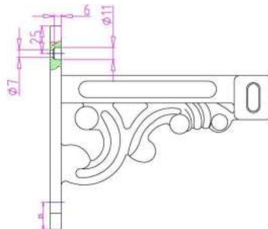
Figura nr. 2 (element fontă partea de jos)
