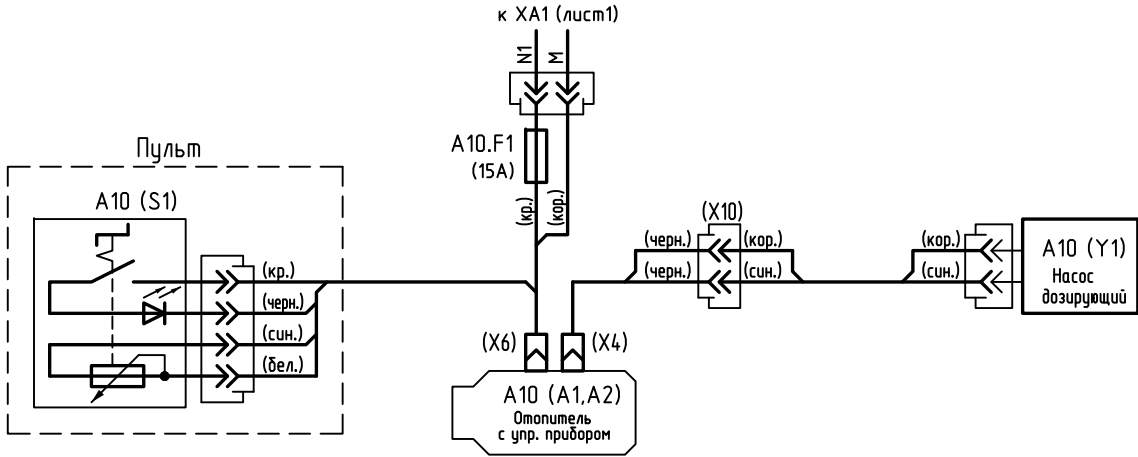
Схема подключения отопителя автономного воздушного Air Top 2000ST D,24В (А10) в кабине крановщика
