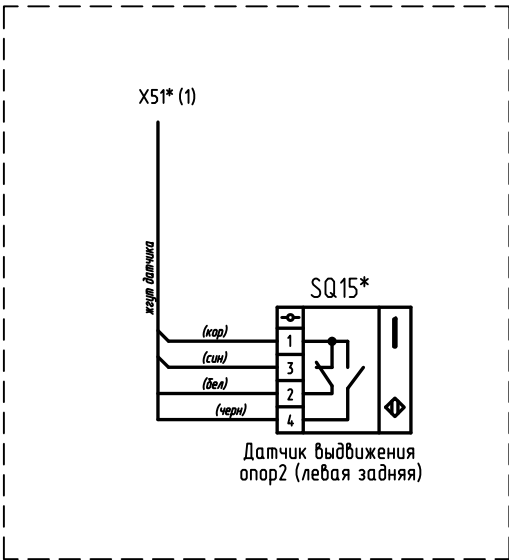
Схема подключения датчика (кран с люлькой)
