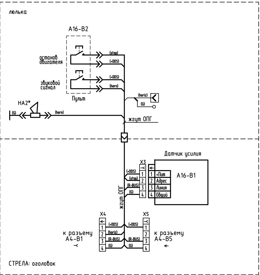
Схема подключения ограничителя предельной грузоподъемности (ОПГ) А16* (кран с люлькой)
