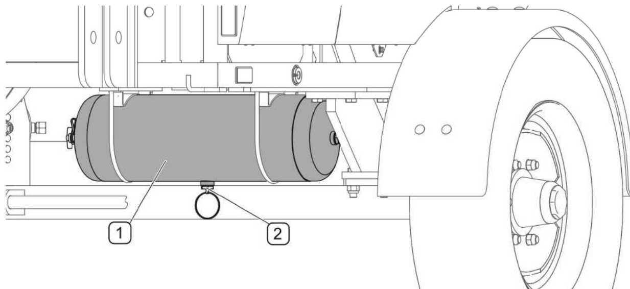
РИСУНОК 5.27А Воздухооборник с конденсатоотводящим клапаном
