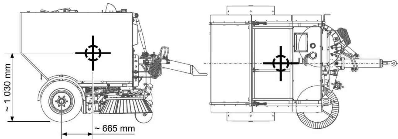
РИСУНОК 1.4А Расположение центра тяжести
