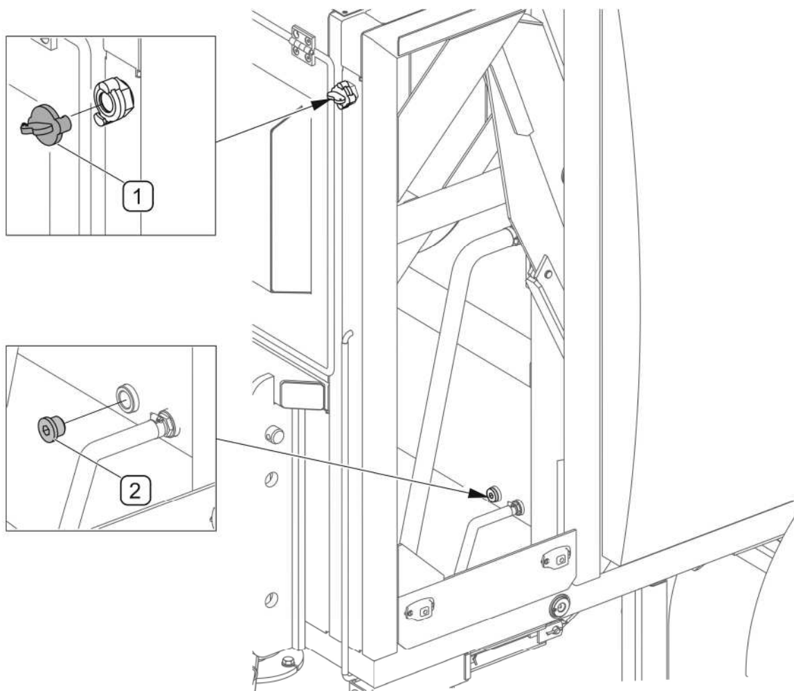
РИСУНОК 5.35А Слив воды из системы полива
