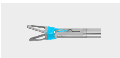
340 mm Ø 5 mm
