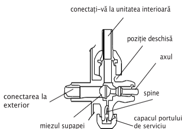
Diagrama supapei cu 3 căi
