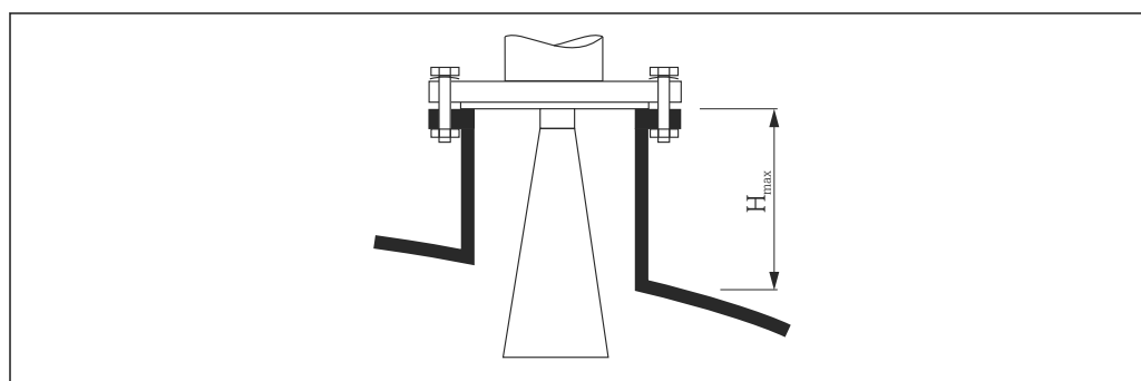
21 Высота патрубка для рупорной антенны (FMR51)
