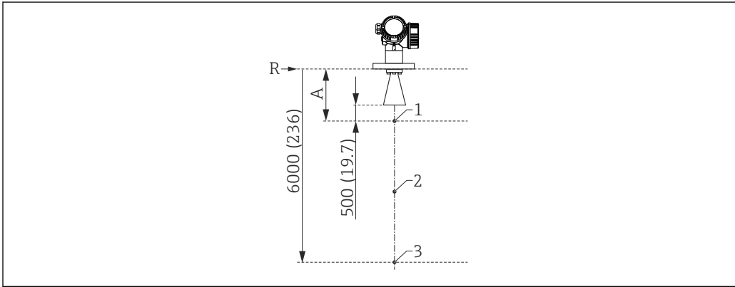
48 Точки калибровочного протокола по 3 точкам; единица измерения: мм (дюймы)
