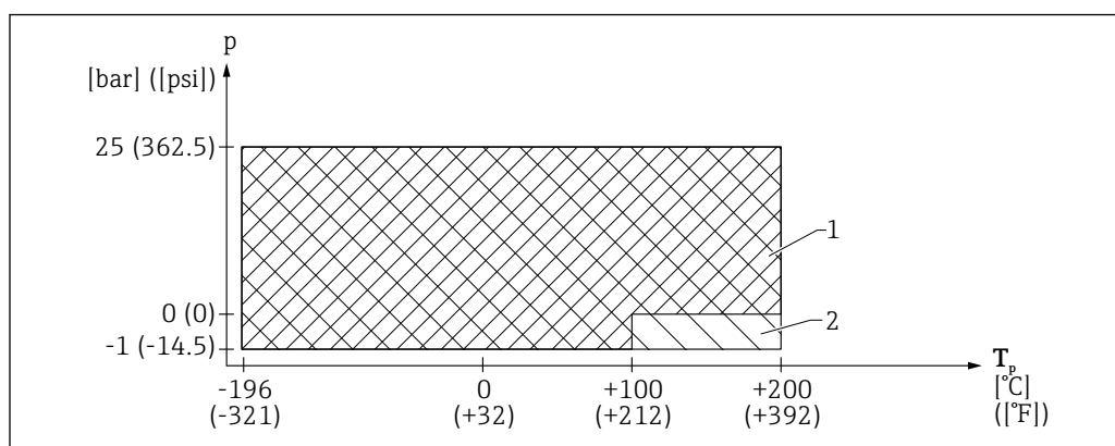
27 FMR52: допустимый диапазон рабочей температуры и рабочего давления
