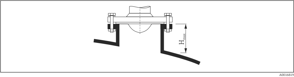
22 Высота патрубка для рупорной антенны, смонтированной заподлицо (FMR52)
