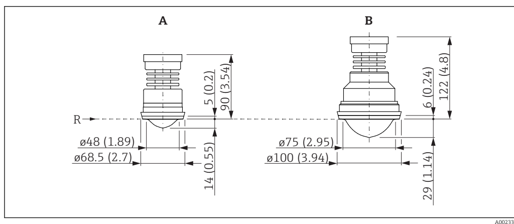
35 Размеры прибора с соединением для молочной трубы согласно стандарту DIN 11851. Единица измерения мм (дюйм)
