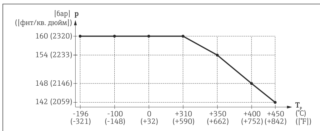
26 FMR51: допустимый диапазон рабочей температуры и рабочего давления для исполнения HT (поз. 090 «Уплотнение», опция D2)
