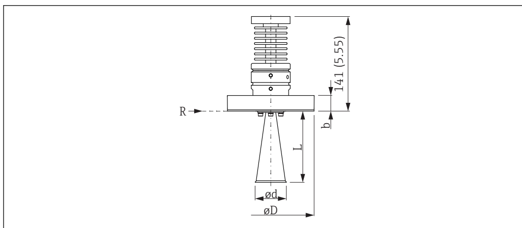
34 Размеры антенны, исполнение для T < 450\text{ °C} (842 °F). Единица измерения мм (дюйм)
