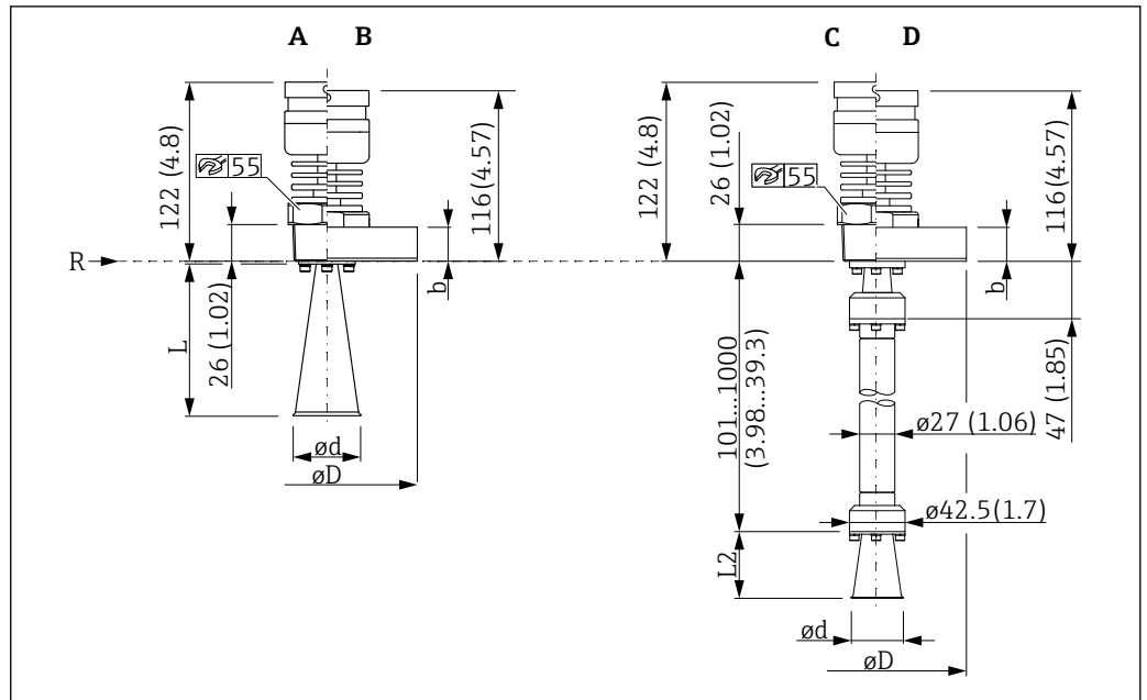
33 Размеры антенны, исполнение для T < 250\text{ °C} (482 °F). Единица измерения мм (дюйм)
