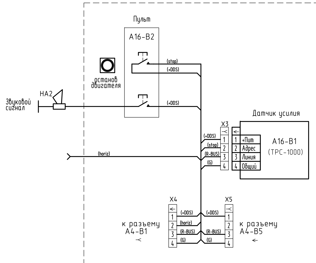
Схема подключения ограничителя предельной грузоподъемности (ОПГ) А16* (кран с люлькой)
