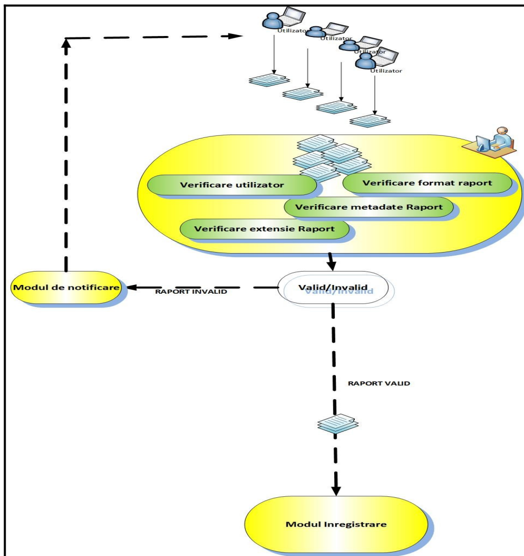
Figura 6. Schema Modului de Validare
