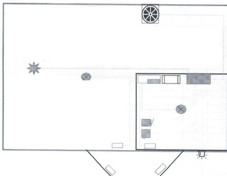
Схема блок- бокса хроматографа
