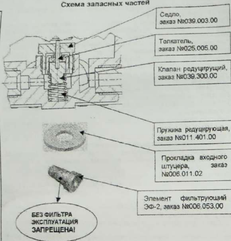
Схема запасных частей
