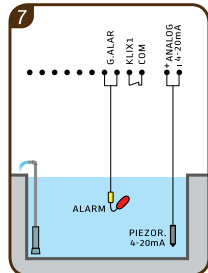
4-20mA mètres
