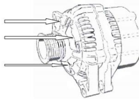
Рис 12.2.3 Місця та напрямок продування стисненим повітрям генератора
