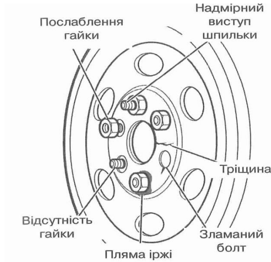
Рисунок 12.7.2 – Надійність встановлення коліс
