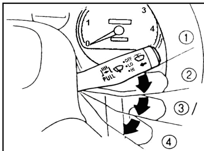
Рисунок 5.3.2 – Положення перемикача склоочисника
