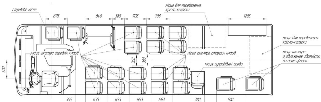
Рис. 3.1 - План салону автобуса D093S4 з двома місцями для школярів з обмеженою здатністю до пересування, решту дивись Рис. 3
