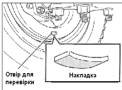
Рисунок 12.7.1.6– Перевірка зношеності гальмівних накладок
