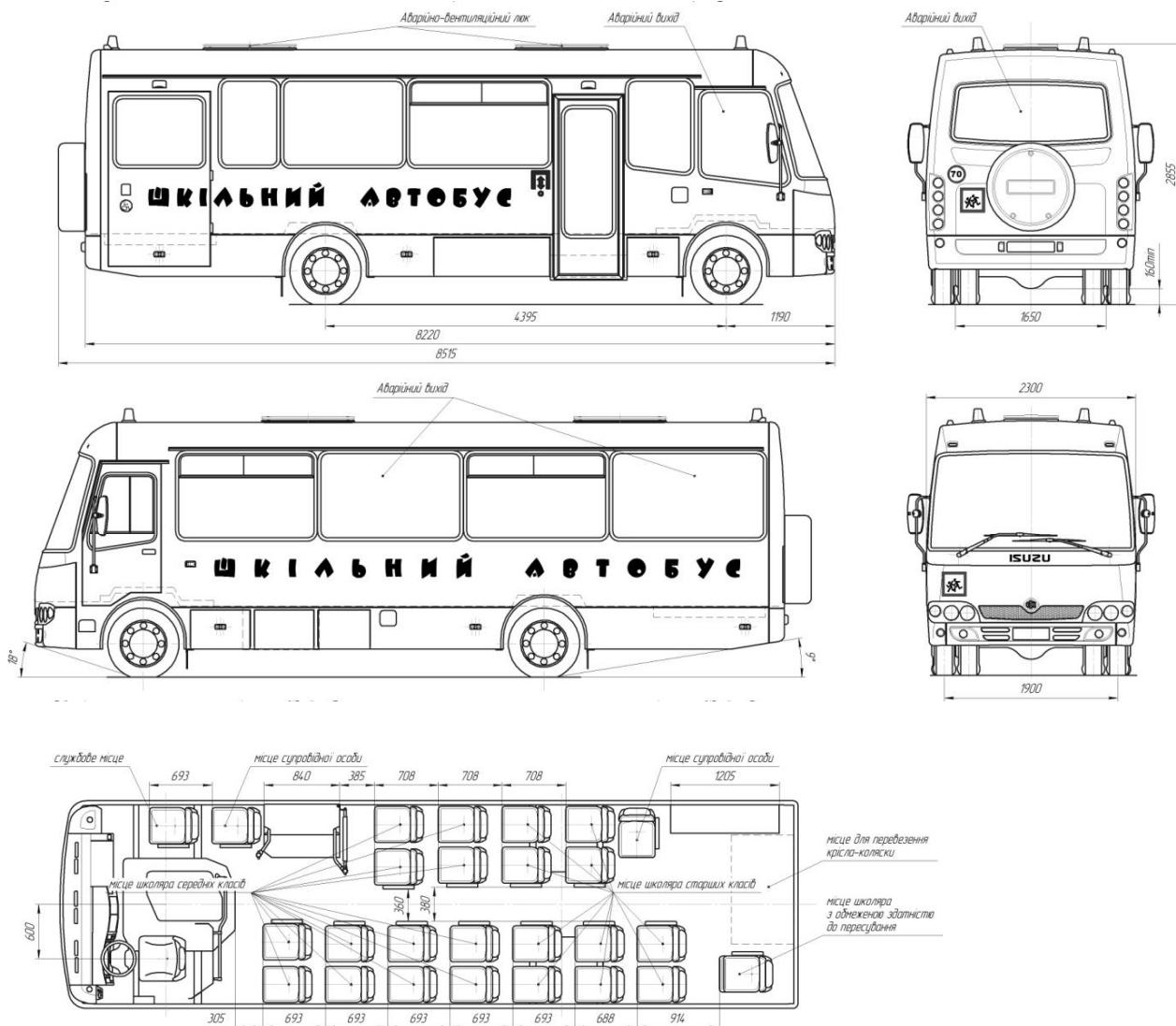
Рис. 3 - Загальний вигляд та план салону автобуса D093S4 з одним місцем для школяра з обмеженою здатністю до пересування.
