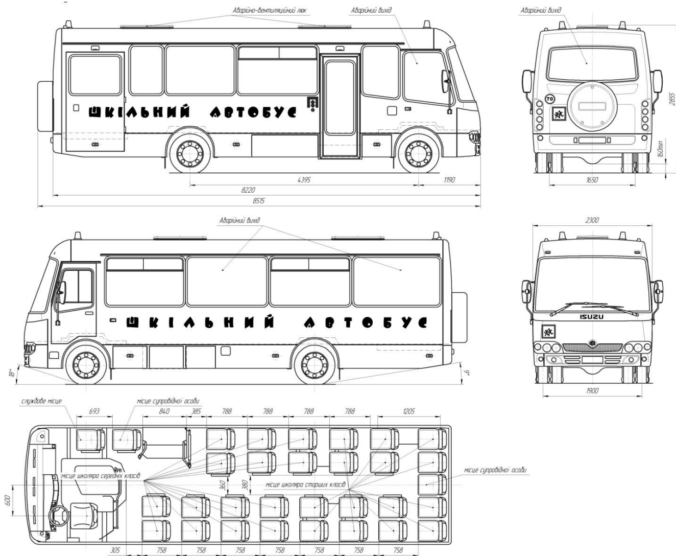
Рис.1 - Загальний вигляд та план салону автобуса D093S2
