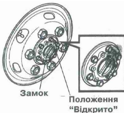
Рис. 5.5.1 Замок маточини в положенні «FREE» (відкрито)
