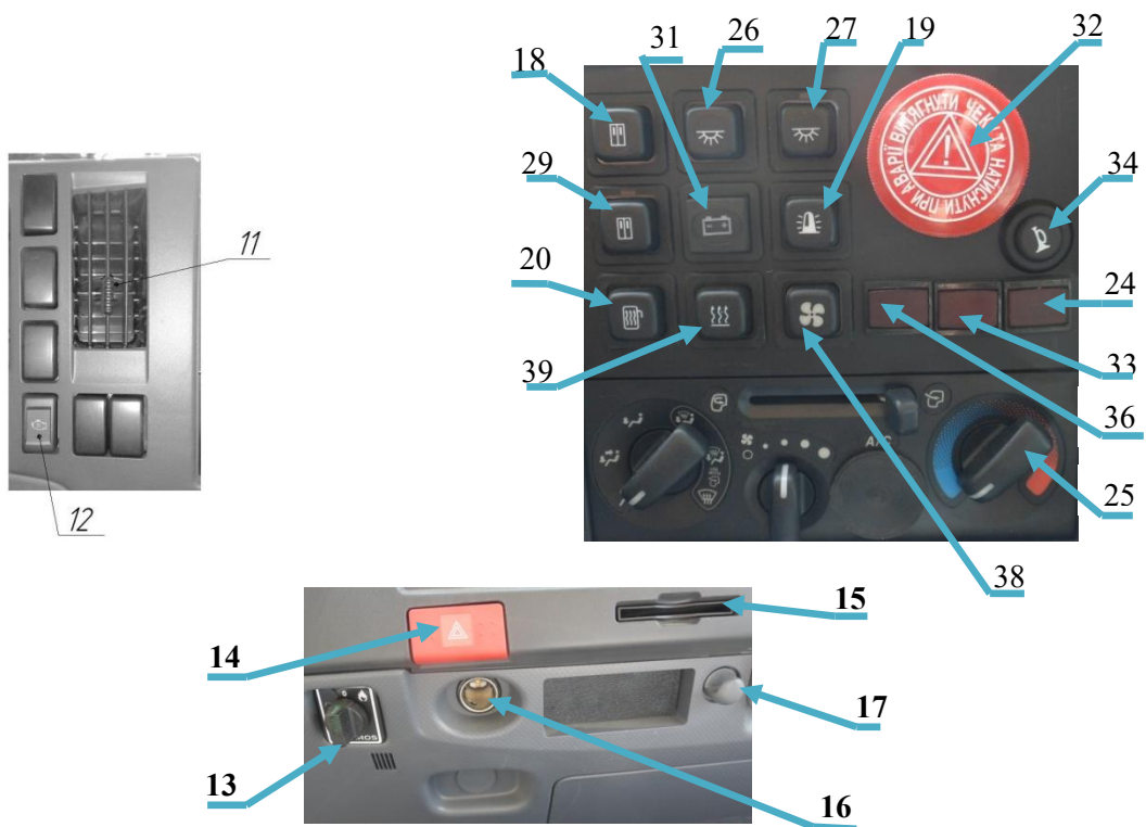
Рисунок 5.1.2 – Основна панель приладів. Ліва частина
