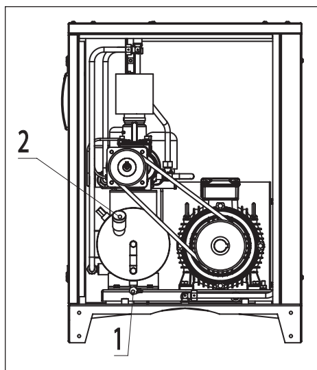
Рис. 5.4.1. Замена масла
