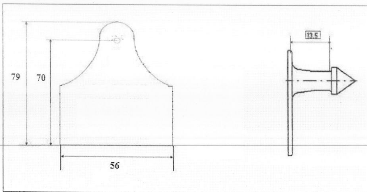
Fig.1 Desen tehnic crotalie neimprimată bovine
