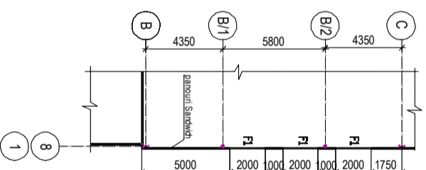
1 - 1 cota 3.500
