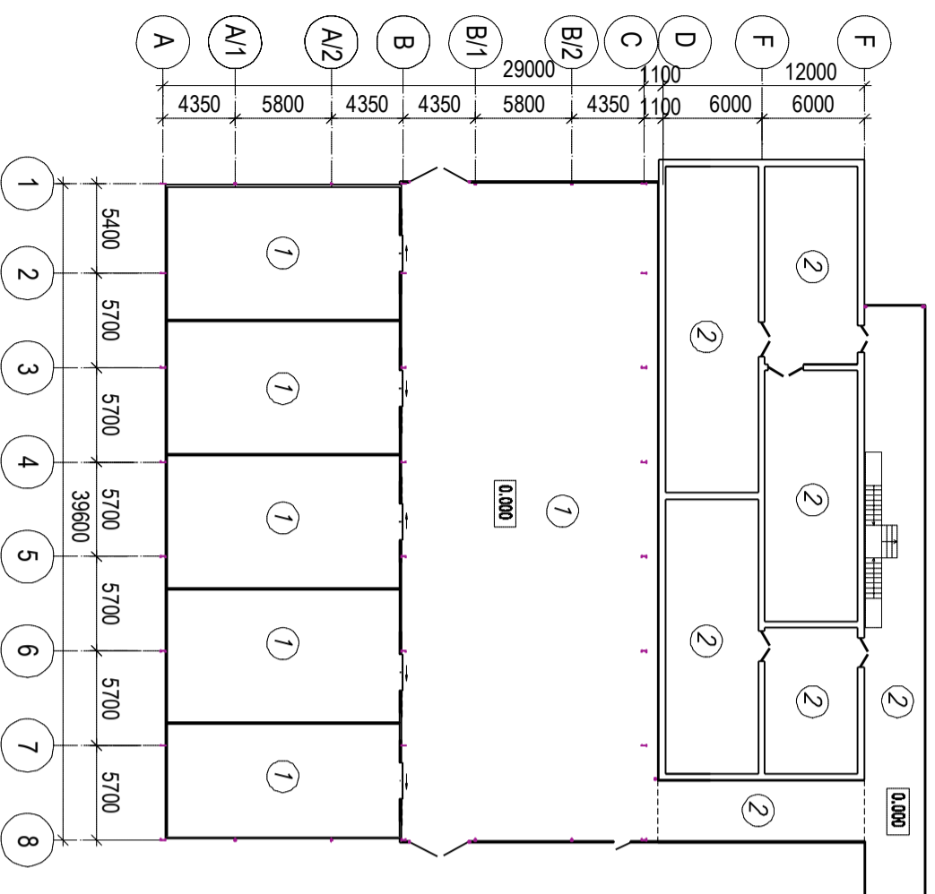
Plan pardosea cota 0.000
