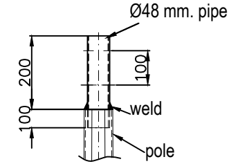
DETAY-C
