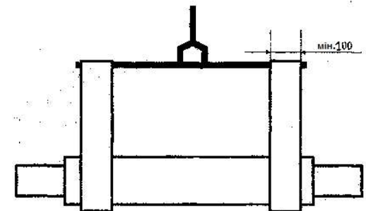
Рис.8. Строповка с помощью мягких полотенец.
