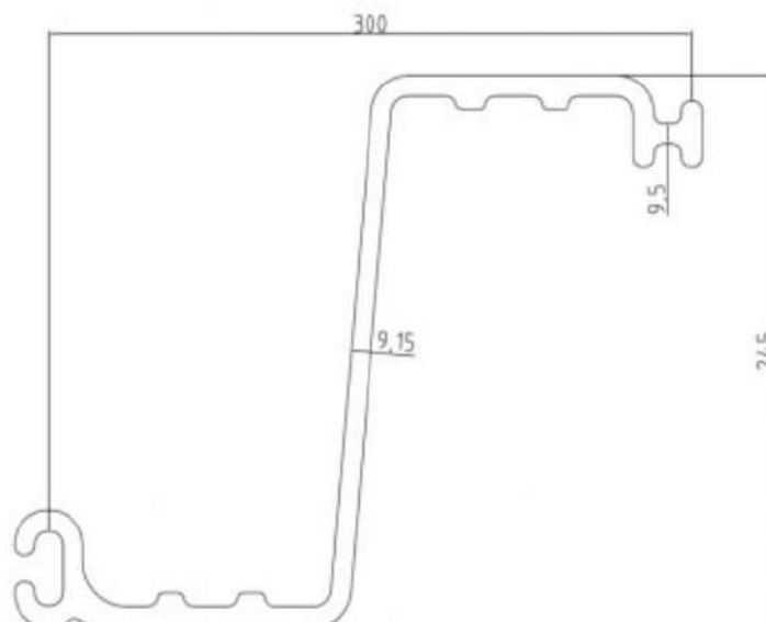
Figura 1 Sectiune palplansa sintetice GW-630-9
