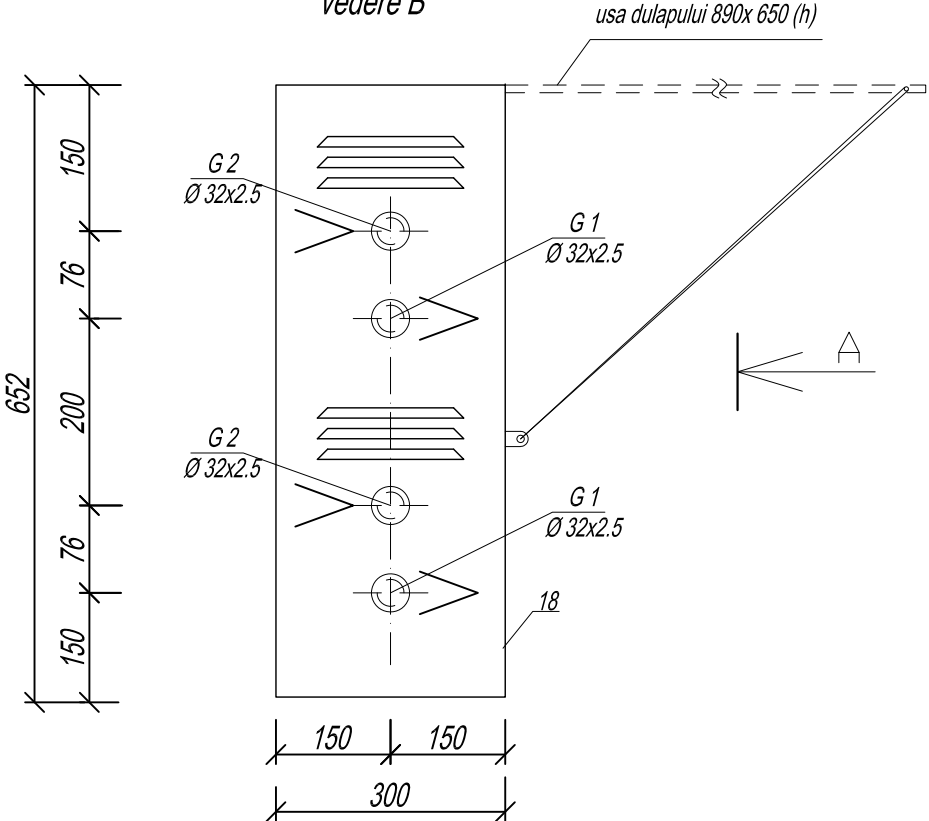
DULAPUL S 1:10 vedere B
