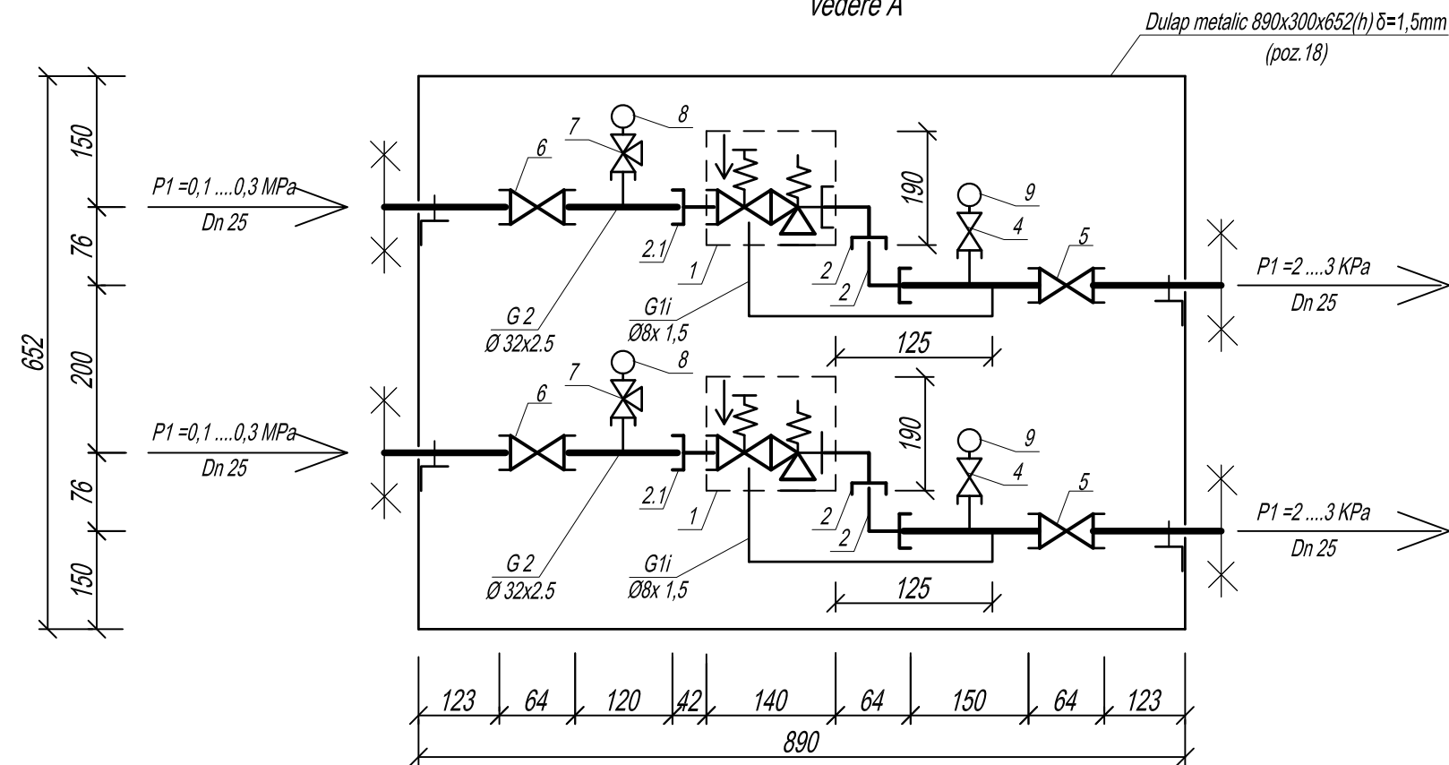
SCHEMA TEHNOLOGICĂ S 1:10 vedere A
