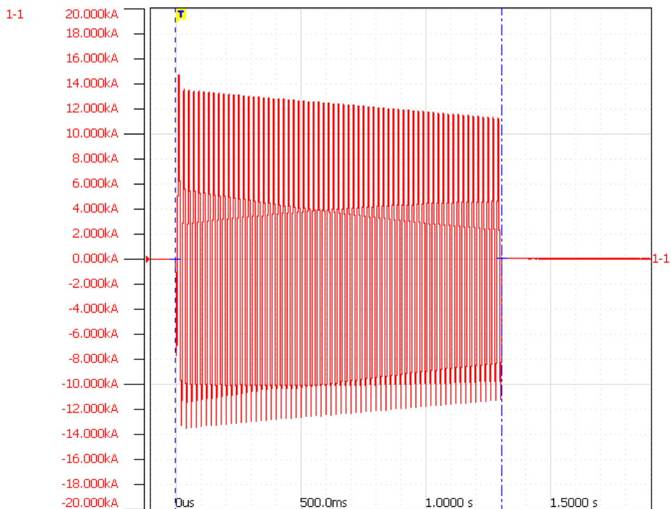
Oscylogram 2. Przebieg prądów podczas próby wytrzymałości zwarcia żyły powrotnej. Próba nr 5580/2019.05.08
