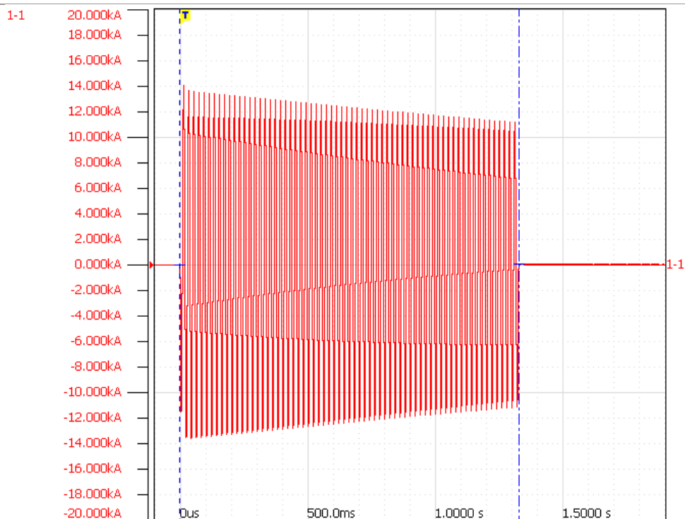
Oscylogram 1. Przebieg prądów podczas próby wytrzymałości zwarcia żyły powrotnej. Próba nr 5579/2019.05.08
