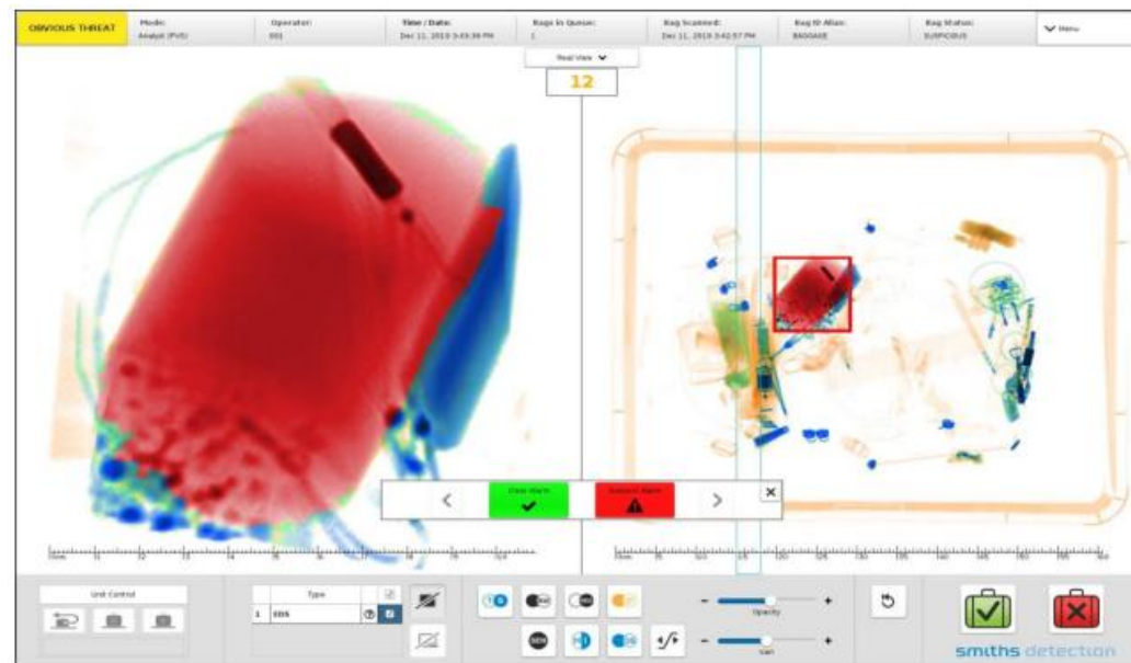
Fereastra de alarmă
