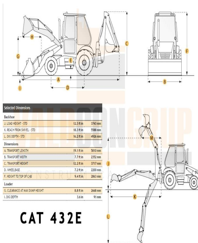
Figura 4. Caracteristicile tehnice CAT432E
