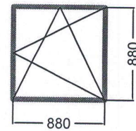
Ferestre 10 buc
