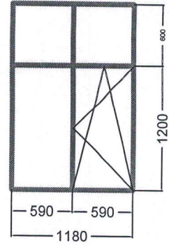
Ferestre 8 buc
