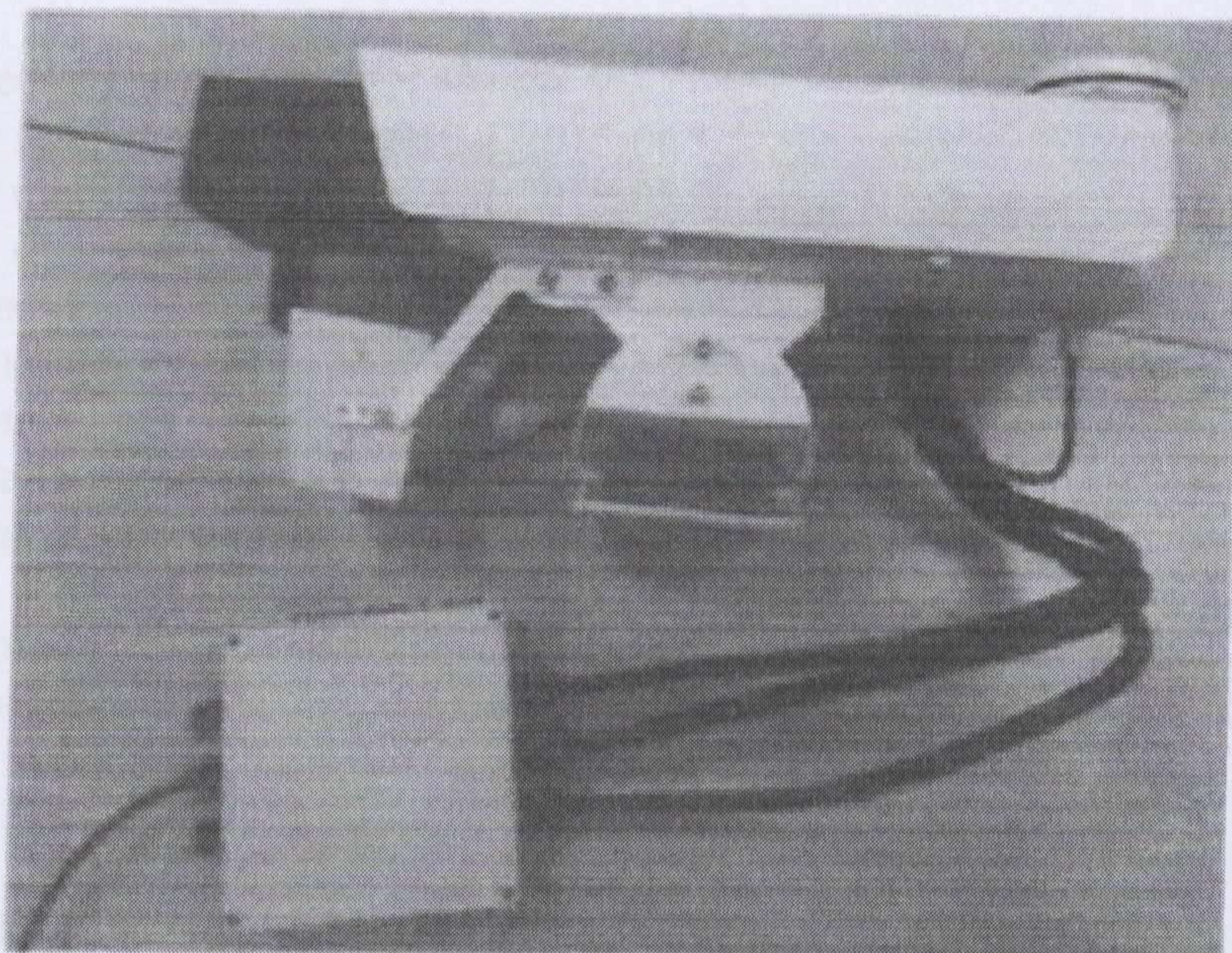
Рис.1. Система измерения скорости «ИТС EYE Compact 300»
