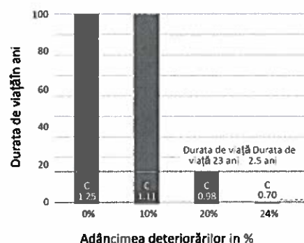
Diagrama duratei de viață în funcție de adâncimea deteriorărilor
