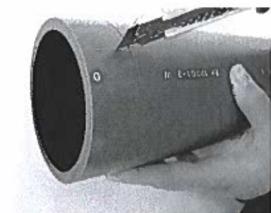
Cu un cutter faceți o tăietură pe cercul stratului superior
