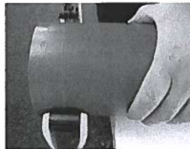
Cu mișcare circulară ușoară, tăiați stratul exterior din PP
