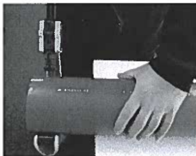
Așezați instrumentul de tăiere în poziție pentru tăiere
