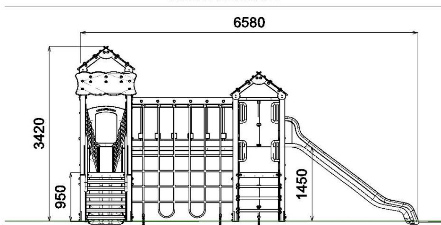
VISTA FRONTALE
