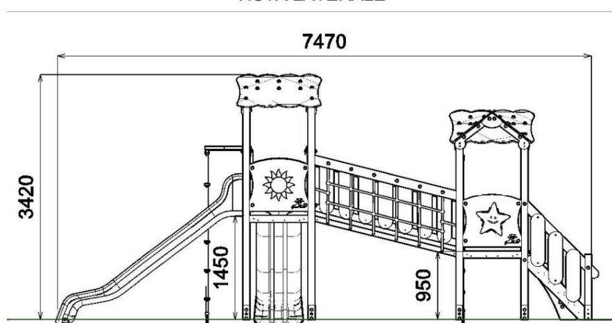
VISTA LATERALE
