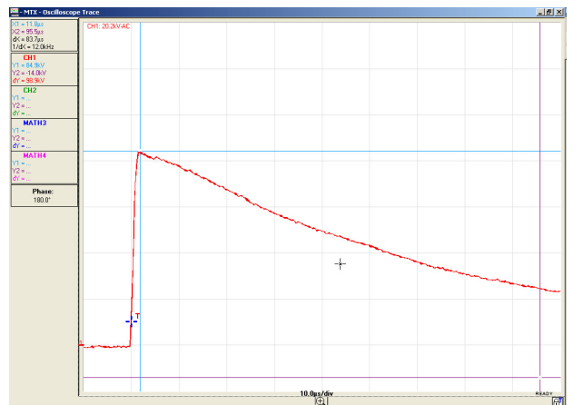
10-й імпульс, U_{test} = 75,0 \text{ кВ}
