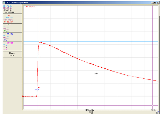
10-й імпульс, U_{test} = 75,1 \text{ кВ}
