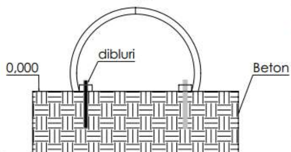
SECTIUNE LA NIVELUL PAMINTULUI 1-2
