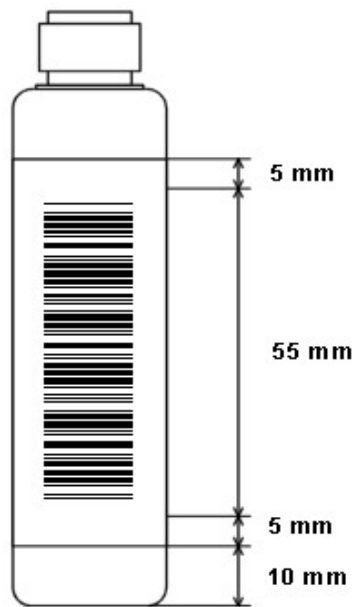
Figură 4.8: Poziționarea etichetei pentru codul de bare al reactivului 1D
