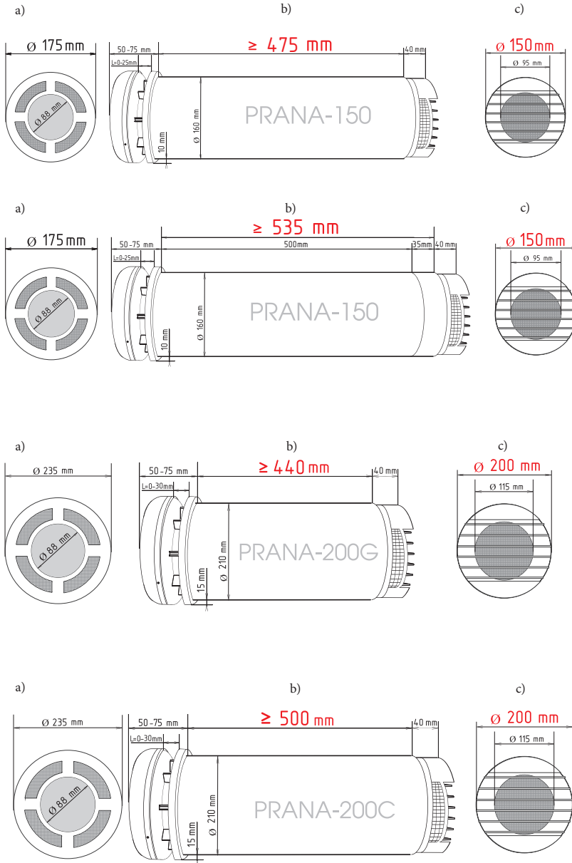
Poza 4. Dimensiunile și schițele recuperatoarelor «PRANA-150», «PRANA-200G», «PRANA-200C»: a) grila de ventilare și admisie din încăpăre; b) unitatea de lucru (lateral); c) grila de ventilare și admisie din exterior.
