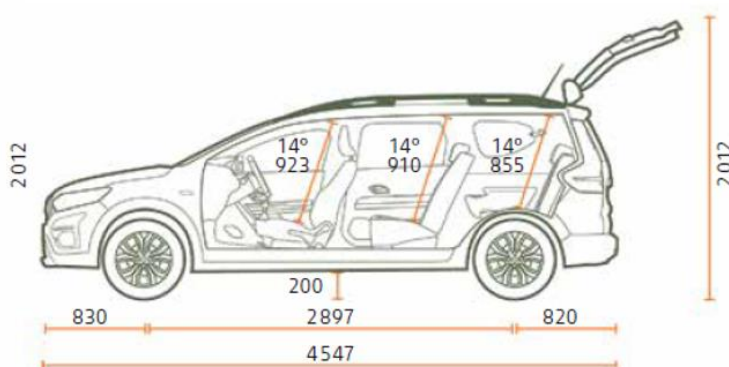
PROFIL 7 LOCURI
