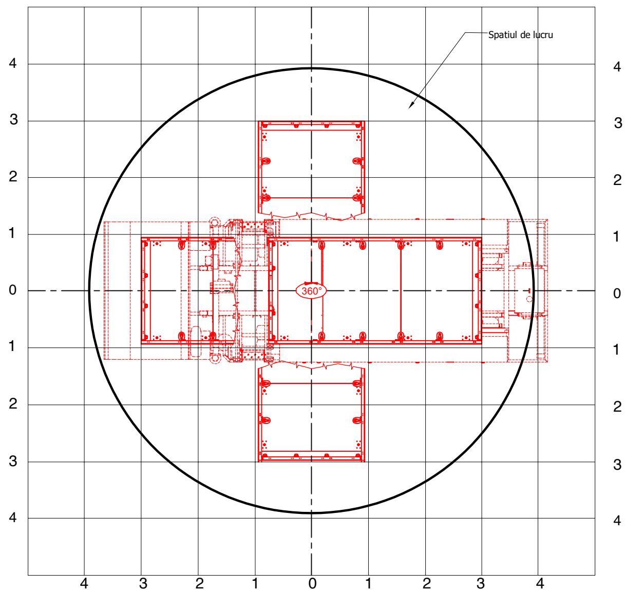
Diagrama de lucru nacela tip foarfeca
