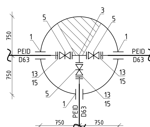
Camin F-58 D1500
