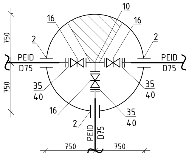
Camin F-50 D1500
