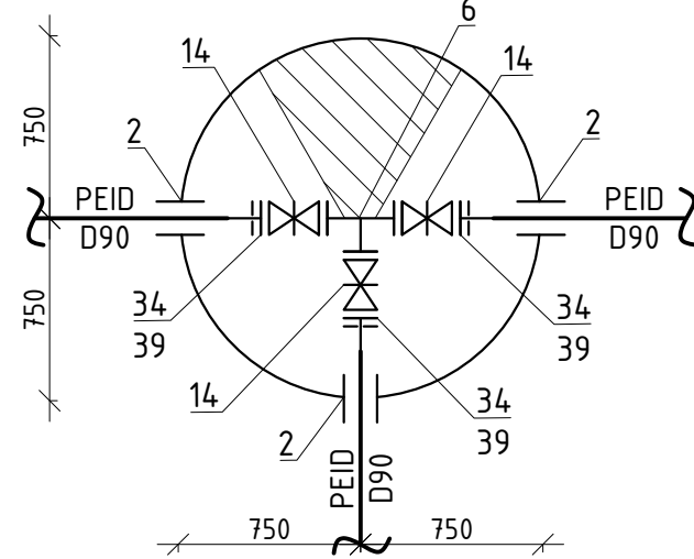
Camin F-25 D1500
