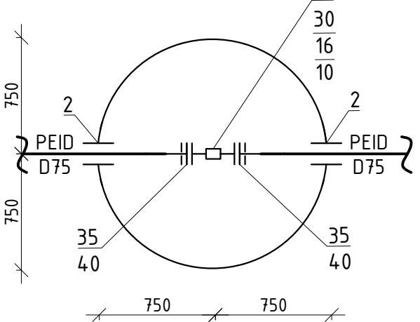
Camin de aerisire CA-23 D1500
