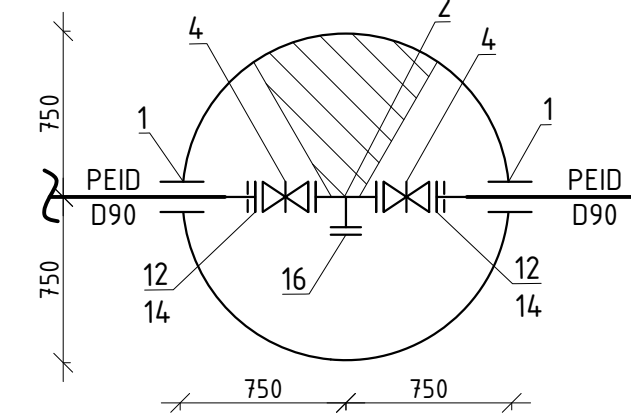
Camin F-31a D1500
