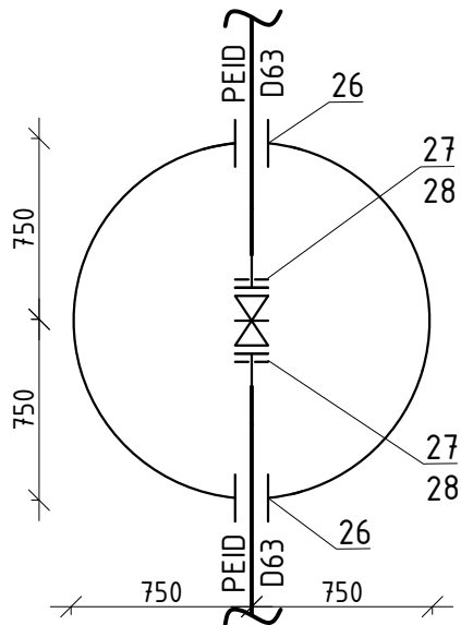
Camin C/VE-11 D1500
