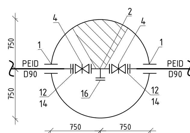
Camin F-61 D1500
