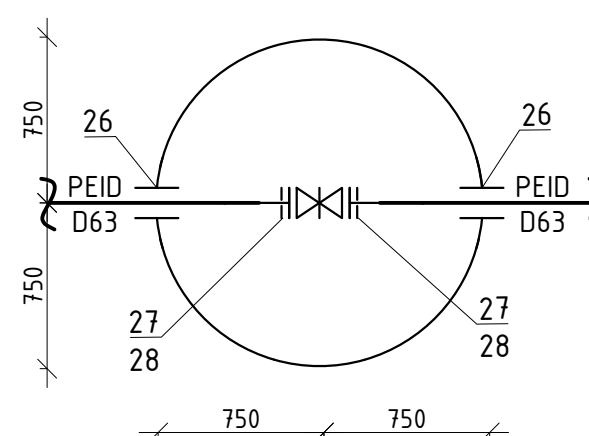
Camin C/VE-8 D1500
