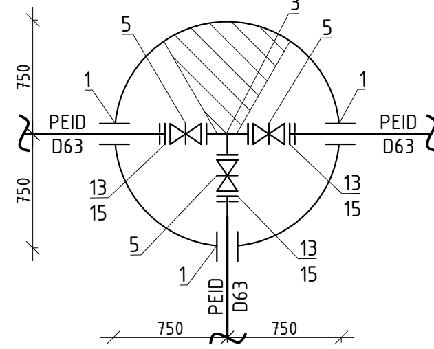
Camin F-28 D1500
