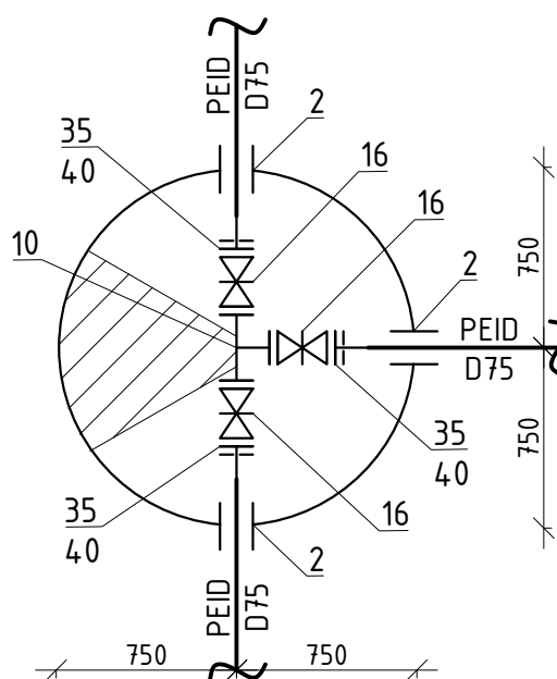
Camin F-14 D1500
