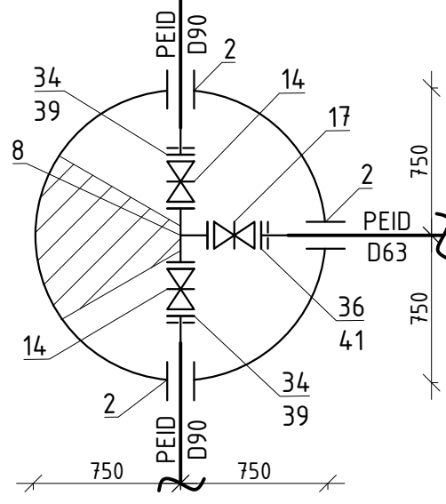
Camin F-26 D1500
