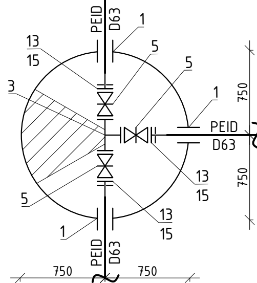
Camin F-27 D1500
