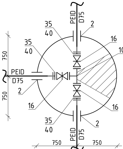
Camin F-16 D1500
