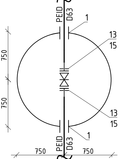
Camin C/VE-3 D1500
