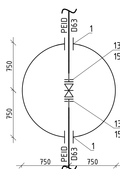
Camin C/VE-9 D1500
