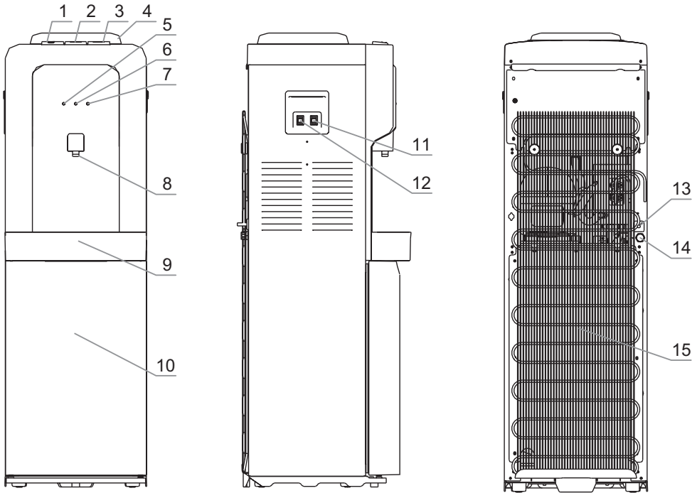
Мал. 1. Схема апарату V900CS
