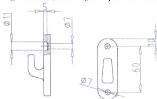
Figura nr. 1 (element fontă partea de sus)
