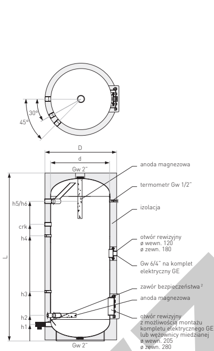
Zasobnik SG(S) Tower Acu 700-1500
