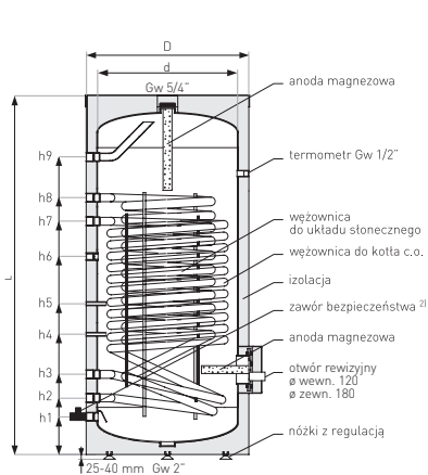
Wymiennik SGW(S)B Tower Biwal Max 200
