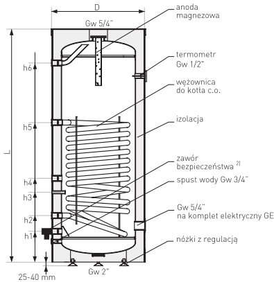
Wymiennik SGW(S) 100-140
