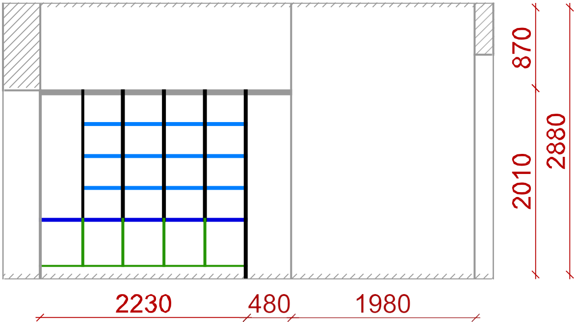
Secțiunea 1-1, Sc.1:40
