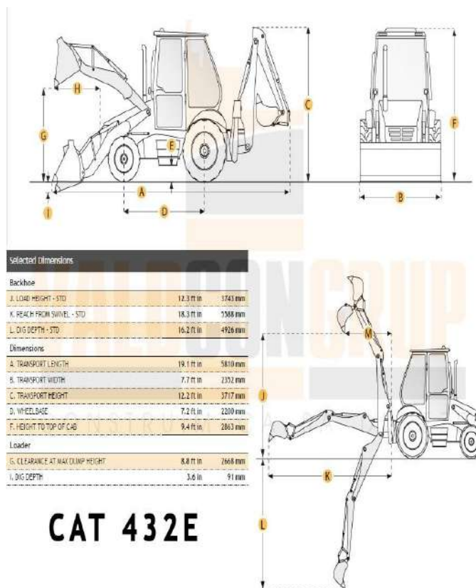
Figura 10. Caracteristicile tehnice CAT432E
