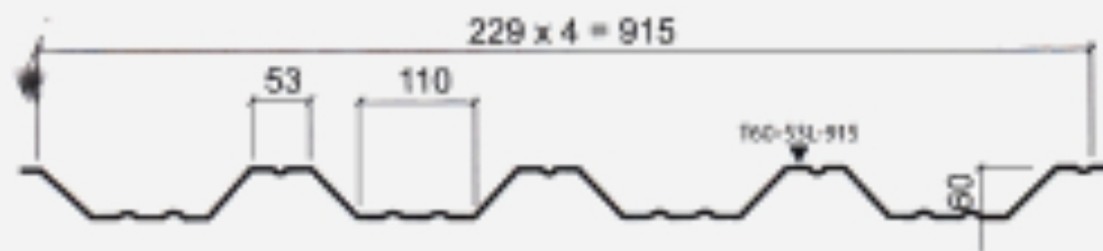
Ruukki T60-53L-915
