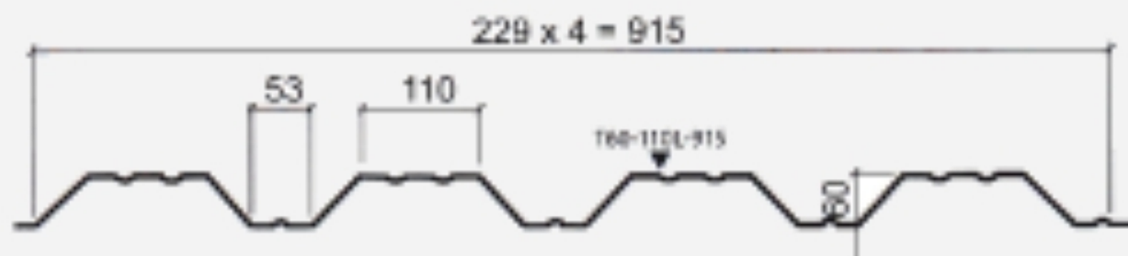
Ruukki T60-110L-915
