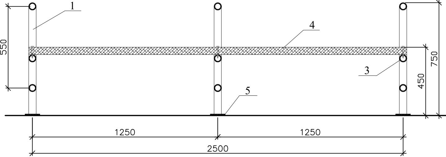
Sectione 1-1
