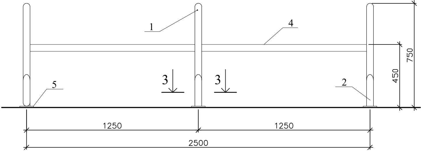
Sectione 1-1
