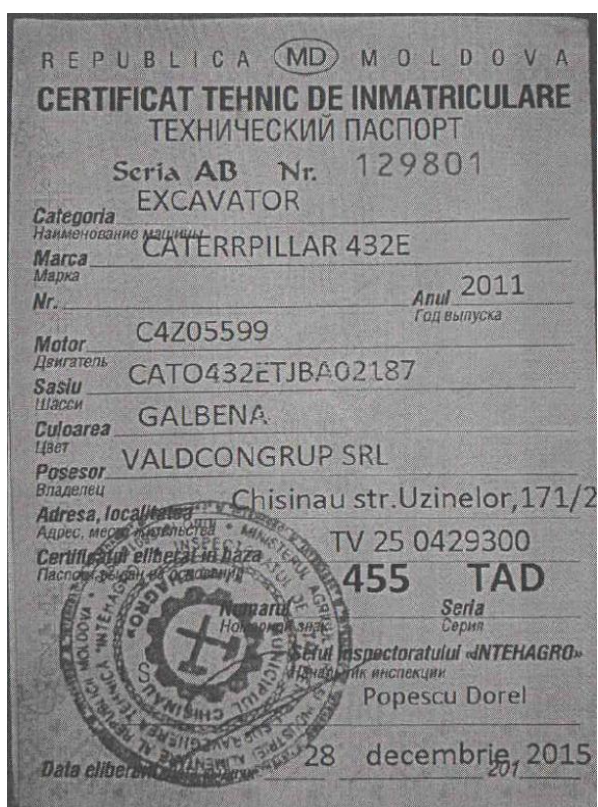
Figura 2. Certificat de înmatriculare CAT432E
