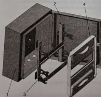
Рисунок 1 – Состав изделия 1 – оболочка, 2 – дверь, 3 – рама монтажная, 4 – панель оперативная
